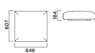
Cushion Module COD. CS10-5095 L648 P607 H184
