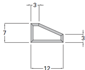
SEZIONE GAMBA LEGNO MDF LEG SECTION PIÈTEMENT EN MDF SECTION
